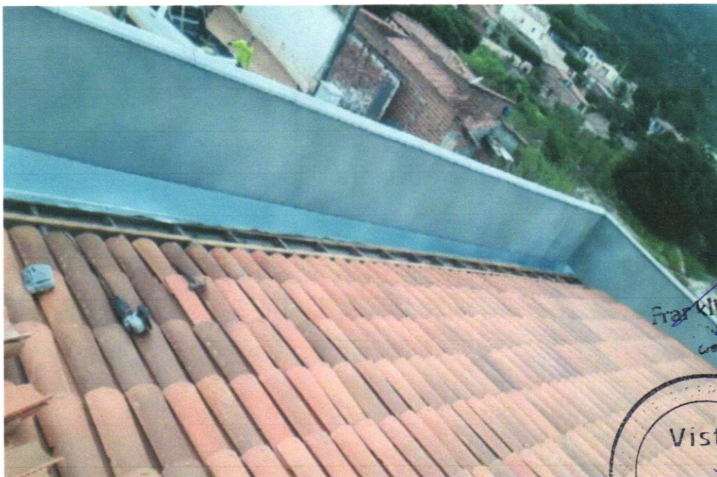
FOTO 08 – Telhamento com telha cerâmica tipo canal, comum, cor vermelha, Itabaiana ou similar
