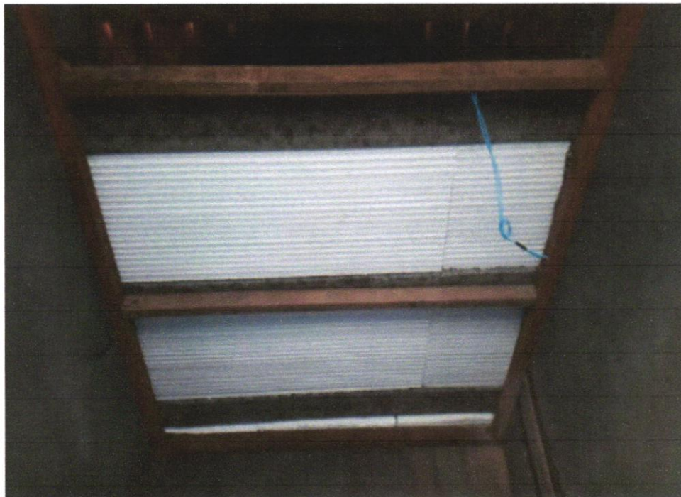
FOTO 11 – Laje pré-fabricada treliçada para piso ou cobertura, intereixo 38cm, h=12cm, el. enchimento em EPS h=8cm, inclusive escoramento em madeira e capeamento 4cm.
